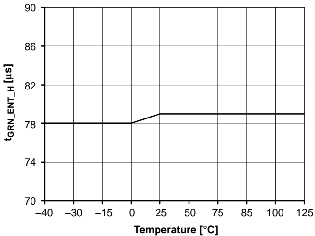
Figure 13. t_{GRN\_ENT\_H}
