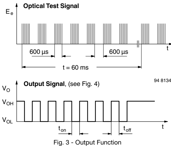
Fig. 3 - Output Function
